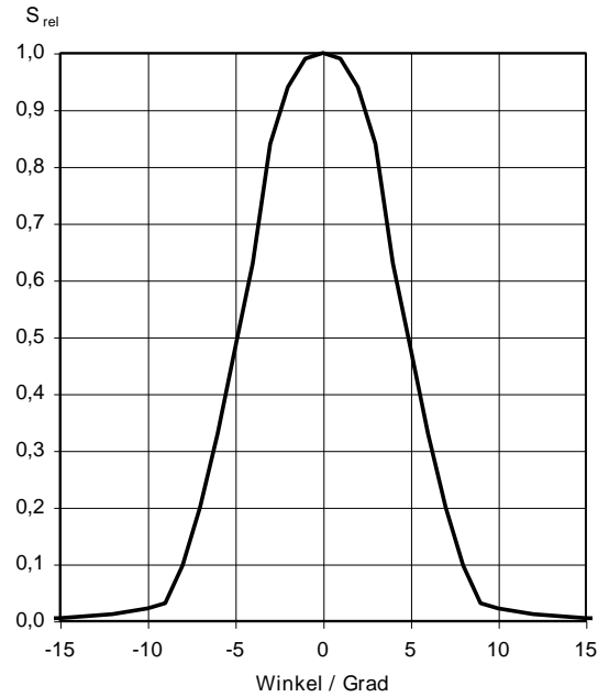
Winkelcharakteristik
